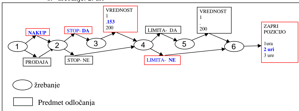
Slika 19: Shema žrebanja parametrov za naključni način trgovanja.
