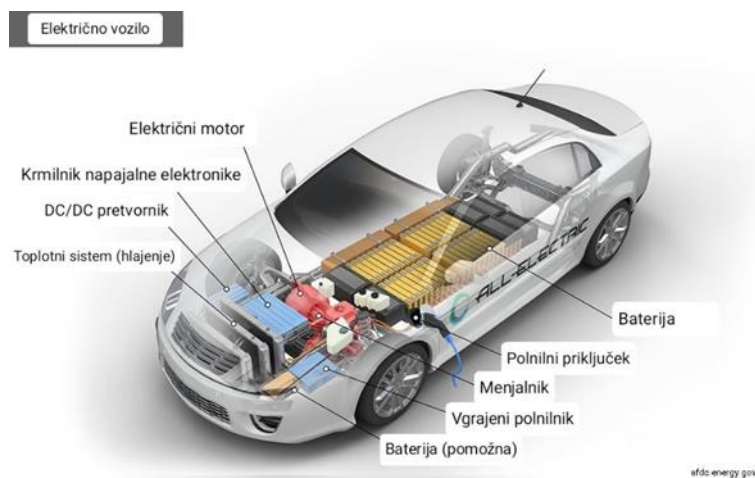
Slika 1: Zgradba električnega avtomobila (1)
