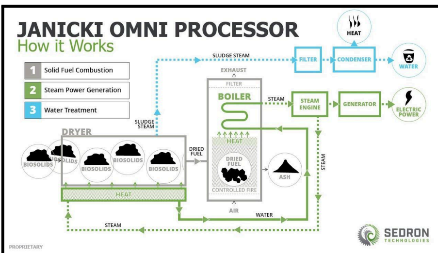
Slika 3: Skica delovanja Janicki omni procesorja.
