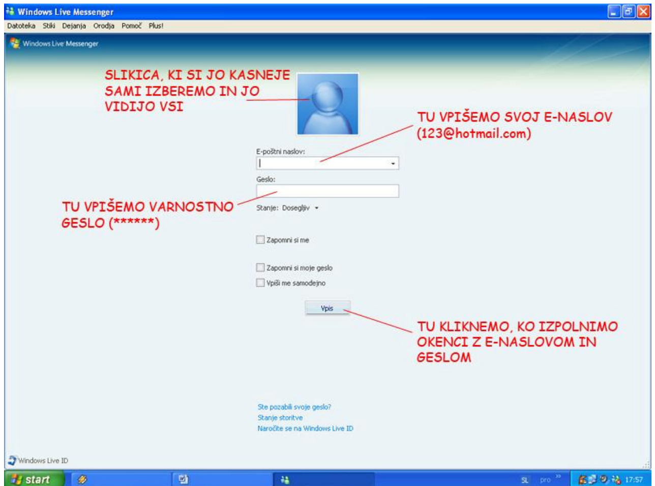
Slika 1: Vpisovalna stran
