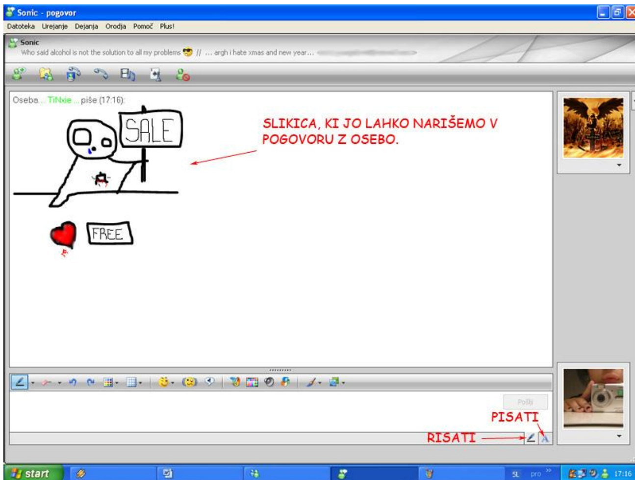
Slika 4: Primer pogovora 2
