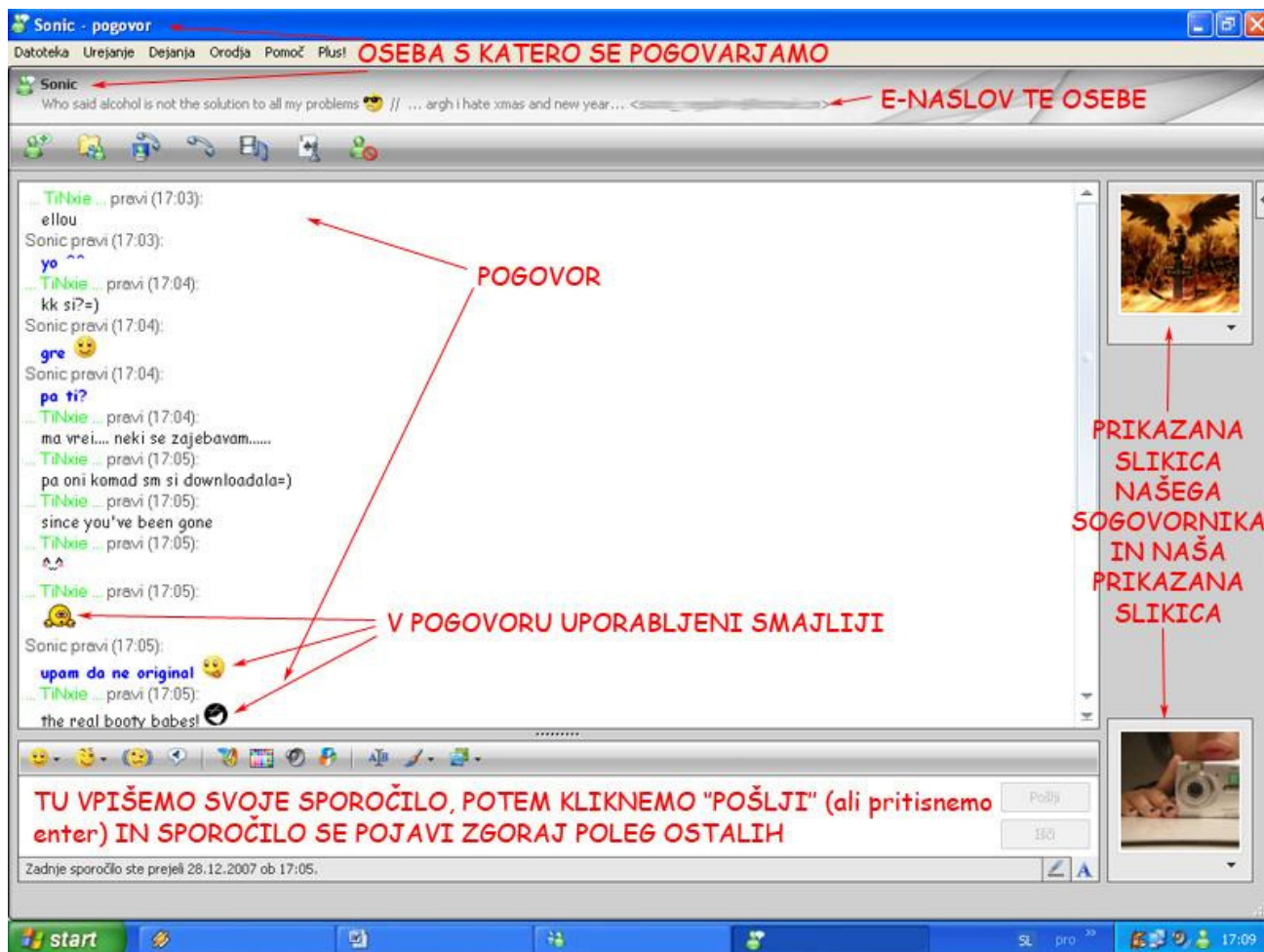
Slika 3: Primer pogovora 1
